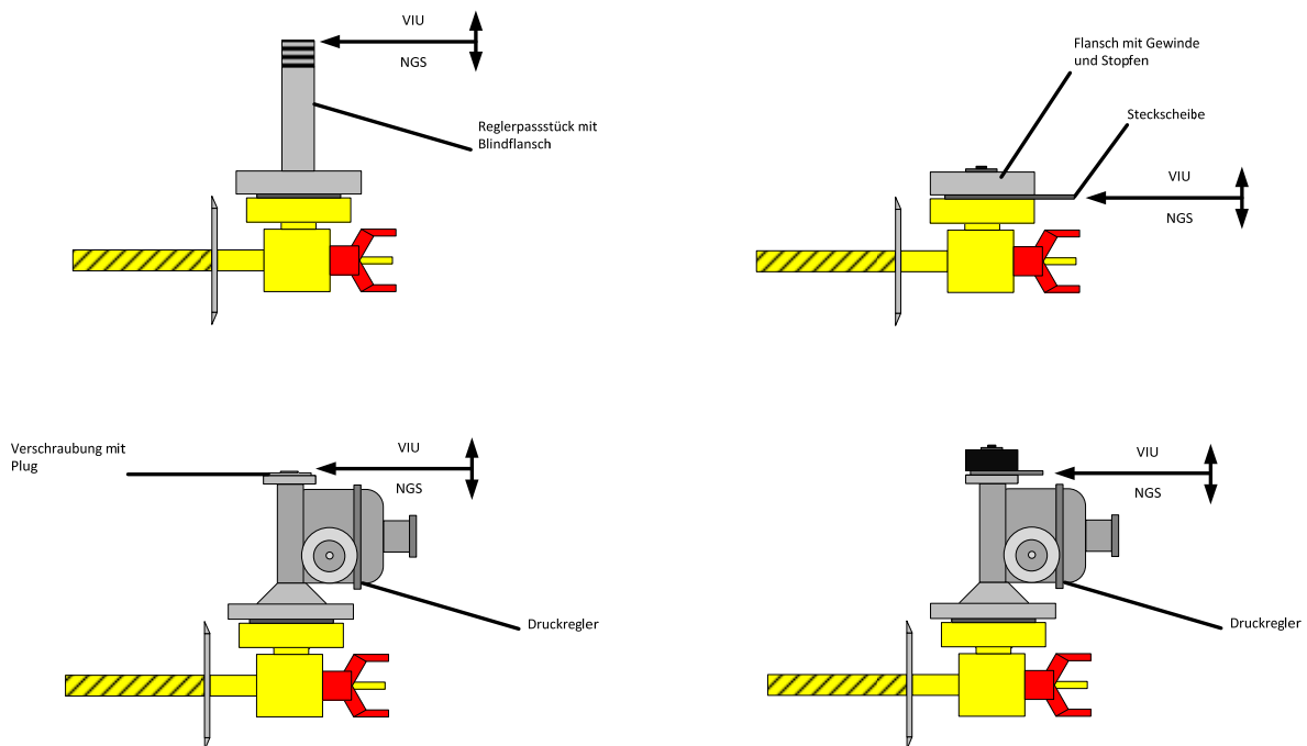
Beispielzeichnungen Eigentumsgrenzen
